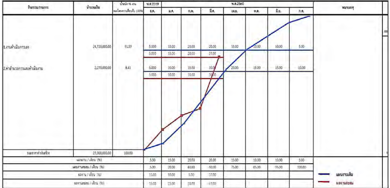
แผน - ควบคุมปริมาณก่อสร้าง โครงการก่อสร้าง สำนักงานเขตพื้นที่ 1 งานก่อสร้างระบบส่งน้ำฝายน้ำแม่เงา (ระยะที่ 2) ตำบลแม่เงา อำเภอขุนยวม จังหวัดแม่ฮ่องสอน ระยะก่อสร้าง มีนาคม 2560
